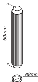
H82 x5
