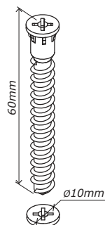
V57 x8
