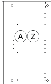
FI10141 676x405x16mm
