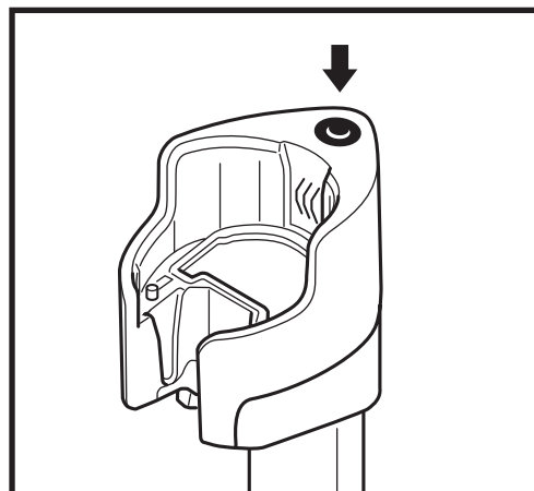
PLACERING AF KNAK FOR QUIET-TILSTAND
