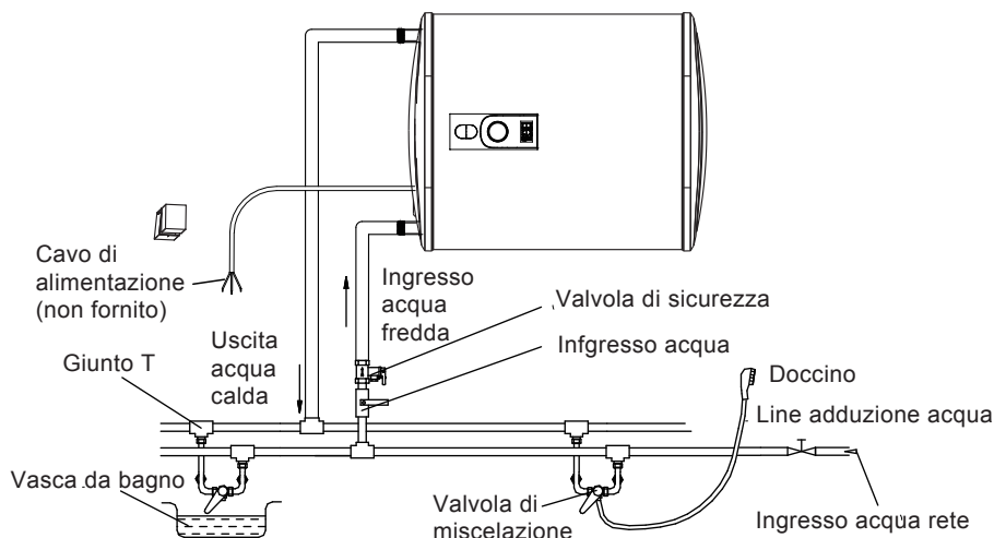
↑ INSTALLAZIONE ORIZZONTALE
